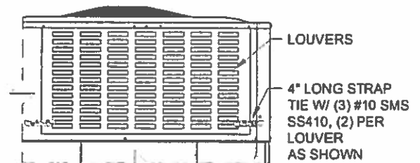
5 LOUVERS REINFORCEMENT SCALE: N.T.S. FRONT VIEW
